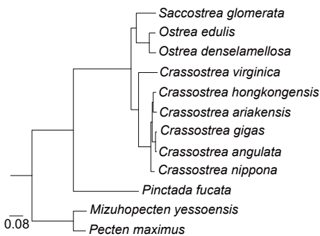
a Ostreida dataset topologies
